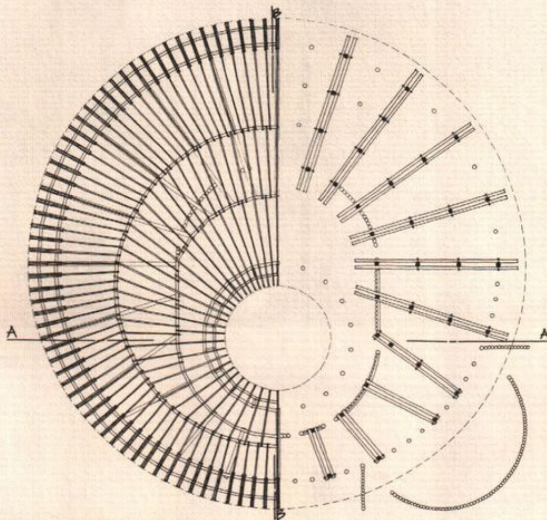
planta de madeiramento
